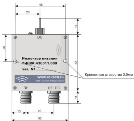
Рисунок – Общий вид изделия.
